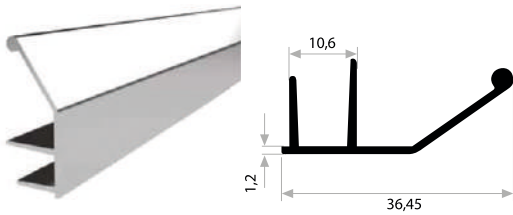
KALIP NO 2003 Kg / m: 0,237
