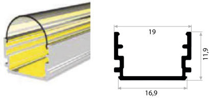
KALIP NO 6003 Kg / m: 0,130
