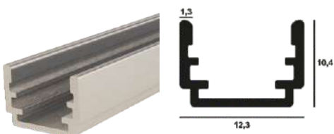
KALIP NO 6012 Kg / m: 0,108
