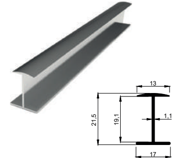
KALIP NO 4052 Kg / m: 0,143
