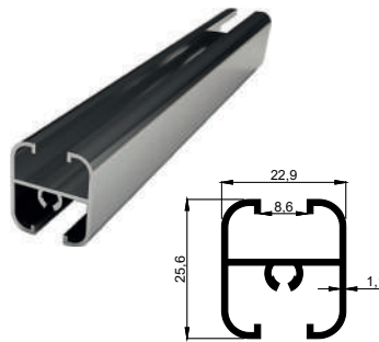
KALIP NO 4085 Kg / m: 0,303
