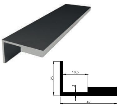
KALIP NO 4022 Kg / m: 0,584
