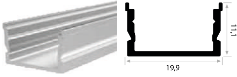
KALIP NO 6001 Kg / m: 0,135
