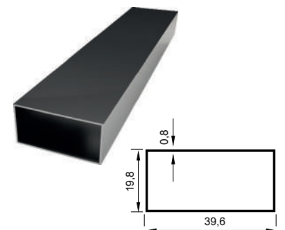
KALIP NO 4116 20x40 Kutu Profil Kg / m: 0,232
