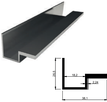
KALIP NO 4003 Kg / m: 0,380
