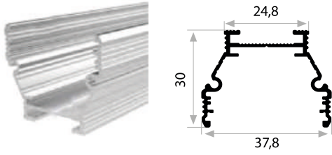
KALIP NO 6011 Kg / m: 0,390
