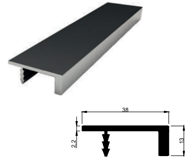
KALIP NO 4029 Kg / m: 0,403
