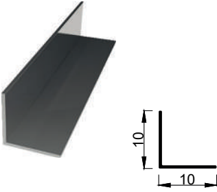
KALIP NO 4122 Kg / m: 0,076
