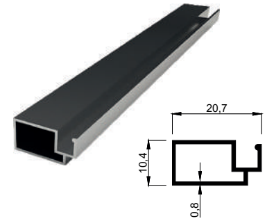
KALIP NO 4113 10x20 Sineklik Kg / m: 0,134
