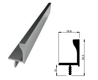
KALIP NO 4035 Kg / m: 0,351
