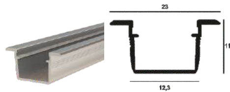
KALIP NO 6008 Kg / m: 0,102
