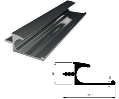
KALIP NO 4026 Kg / m: 0,534
