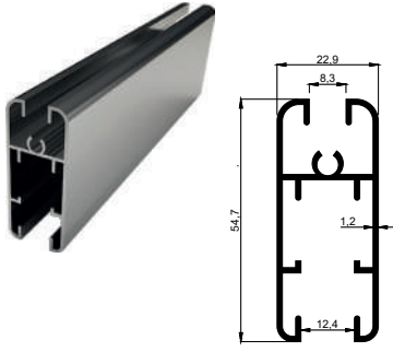
KALIP NO 4081 Kg / m: 0,617
