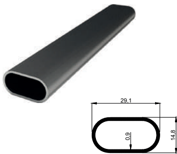
KALIP NO 4102 Kg / m: 0,151
