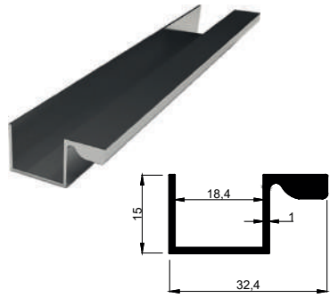
KALIP NO 4004 Kg / m: 0,242
