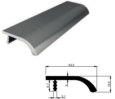
KALIP NO 4030 Kg / m: 0,489
