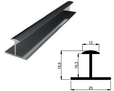
KALIP NO 4049 Kg / m: 0,179
