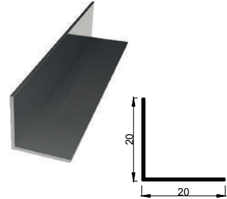
KALIP NO 4124 Kg / m: 0,127
