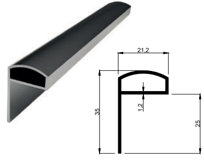
KALIP NO 4119 Kg / m: 0,254
