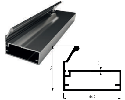
KALIP NO 4101 Kg / m: 0,489
