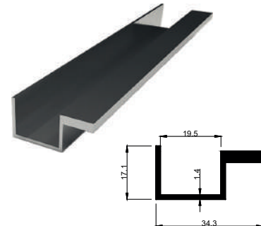
KALIP NO 4007 Kg / m: 0,321
