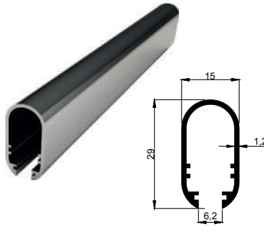
KALIP NO 4121 Kg / m: 0,245
