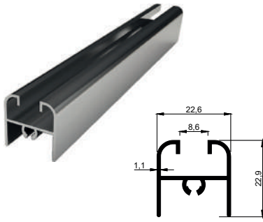
KALIP NO 4084 Kg / m: 0,285
