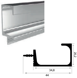
KALIP NO 4027 Kg / m: 0,302
