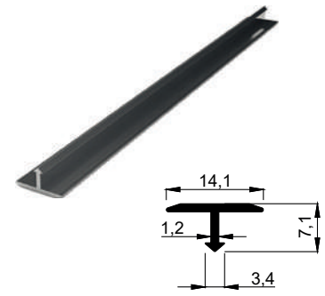
KALIP NO 4055 Kg / m: 0,064
