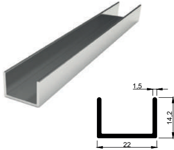
KALIP NO 4042 Kg / m: 0,196
