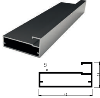
KALIP NO 4094 Kg / m: 0,424
