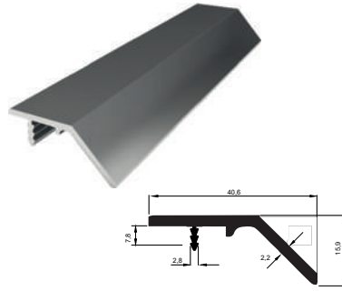
KALIP NO 4028 Kg / m: 0,322
