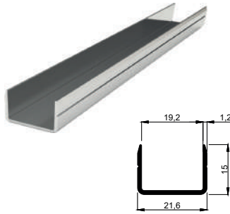
KALIP NO 4040 Kg / m: 0,154
