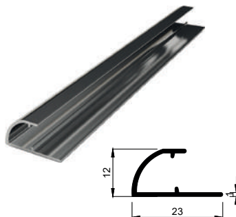
KALIP NO 4091 Kg / m: 0,122
