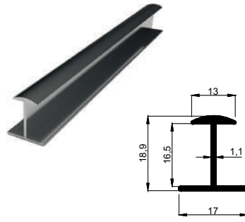
KALIP NO 4048 Kg / m: 0,135
