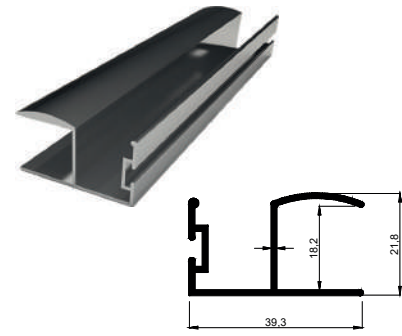
KALIP NO 4020 Kg / m: 0,382
