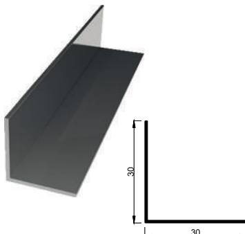
KALIP NO 4126 Kg / m: 0,193
