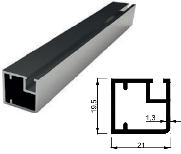
KALIP NO 4093 Kg / m: 0,324
