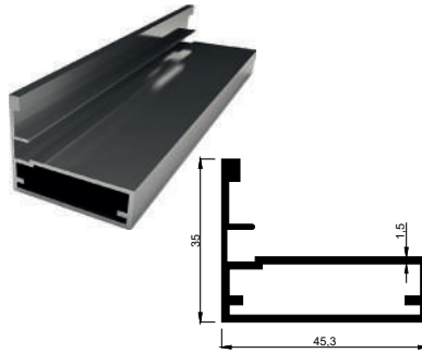
KALIP NO 4100 Kg / m: 0,596
