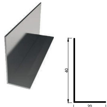
KALIP NO 4127 Kg / m: 0,210
