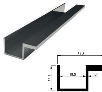
KALIP NO 4009 Kg / m: 0,327
