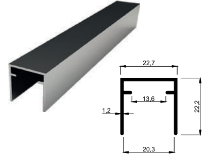
KALIP NO 4072 Kg / m: 0,230
