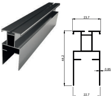
KALIP NO 4114 Plise Kanat Sineklik Kg / m: 0,350
