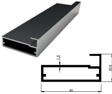
KALIP NO 4096 Kg / m: 0,503
