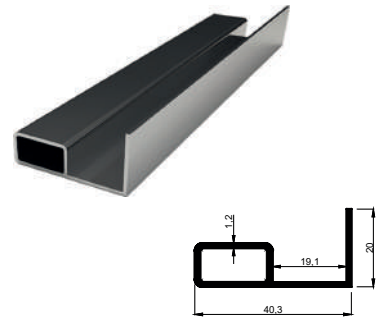
KALIP NO 4014 Kg / m: 0,290
