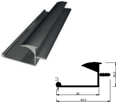
KALIP NO 4024 Kg / m: 0,365
