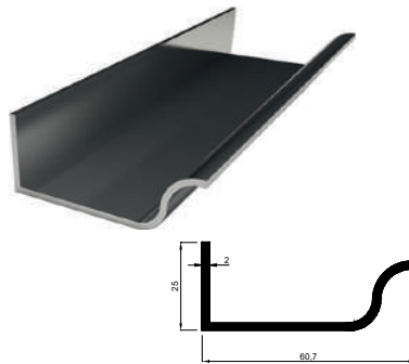
KALIP NO 4019 Kg / m: 0,492
