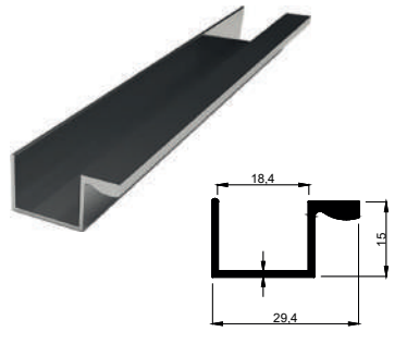
KALIP NO 4005 Kg / m: 0,210
