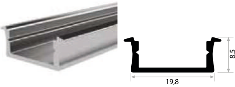
KALIP NO 6005 Kg / m: 0,135
