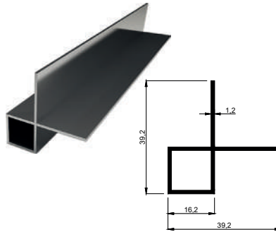
KALIP NO 4076 Kg / m: 0,313
