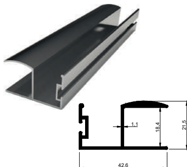
KALIP NO 4021 Kg / m: 0,282
