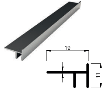
KALIP NO 4095 Kg / m: 0,095
