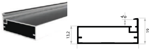
KALIP NO 2001 Kg / m: 0,416
