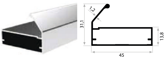
KALIP NO 2005 Kg / m: 0,456
