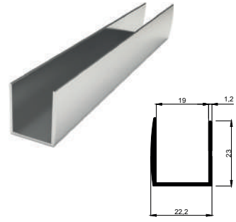
KALIP NO 4038 Kg / m: 0,230
