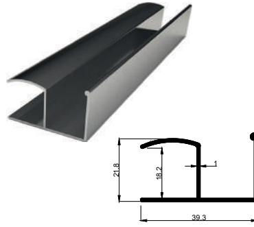
KALIP NO 4001 Kg / m: 0,265
