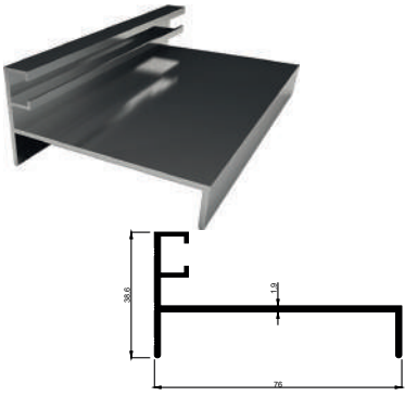
KALIP NO 4073 Kg / m: 0,698
