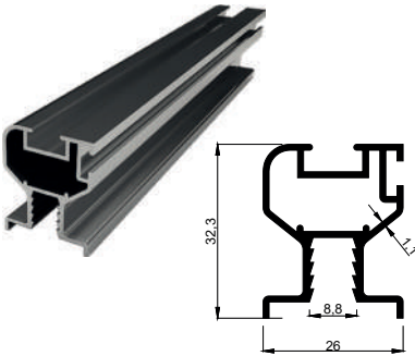
KALIP NO 4087 Kg / m: 0,458
