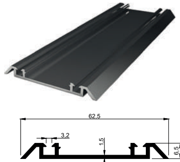
KALIP NO 4082 Kg / m: 0,382
