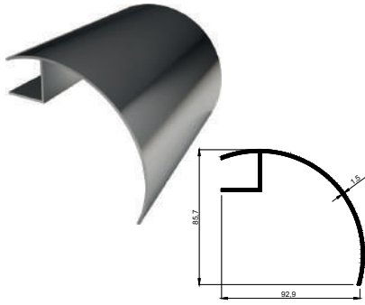
KALIP NO 4012 Kg / m: 0,319
