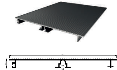
KALIP NO 4044 Kg / m: 0,567
