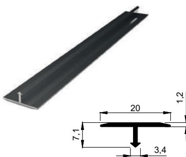
KALIP NO 4056 Kg / m: 0,083
