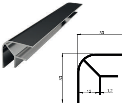
KALIP NO 4079 Kg / m: 0,265
