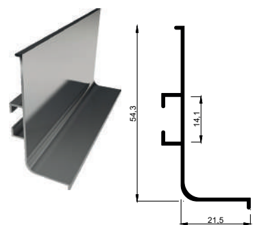
KALIP NO 4033 Kg / m: 0,315
