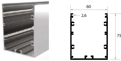
KALIP NO 6013 Kg / m: 1,215
