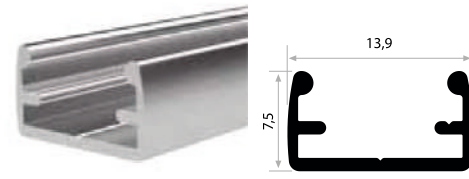
KALIP NO 6006 Kg / m: 0,085
