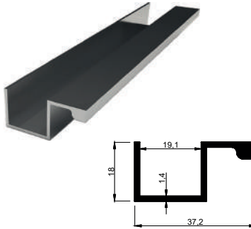
KALIP NO 4006 Kg / m: 0,340
