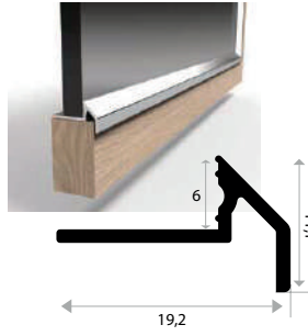
KALIP NO 4097 Kg / m: 0,096
