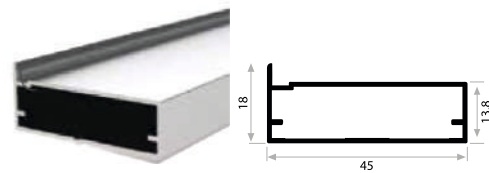
KALIP NO 2004 Kg / m: 0,380
