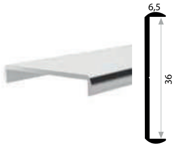
KALIP NO 4039 Kg / m: 0,189
