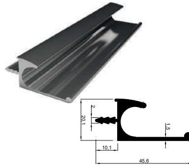
KALIP NO 4025 Kg / m: 0,421
