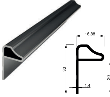
KALIP NO 4118 Kg / m: 0,232
