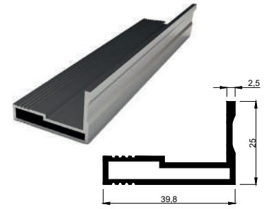
KALIP NO 4098 Kg / m: 0,450
