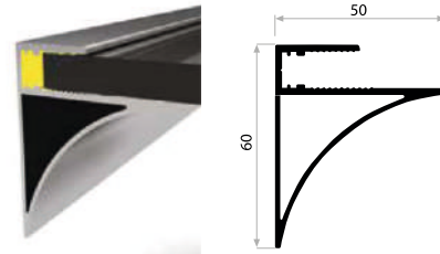
KALIP NO 6014 Kg / m: 0,936
