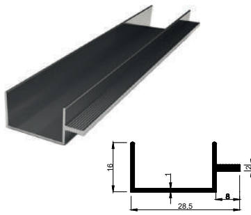
KALIP NO 4016 Kg / m: 0,176
