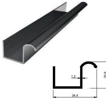
KALIP NO 4013 Kg / m: 0,226
