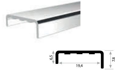
KALIP NO 4041 Kg / m: 0,115
