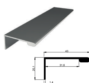
KALIP NO 4023 Kg / m: 0,298
