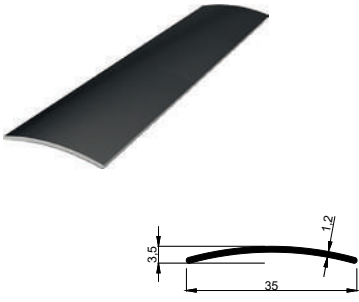
KALIP NO 4105 Kg / m: 0,106
