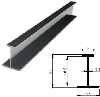
KALIP NO 4053 Kg / m: 0,134
