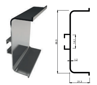
KALIP NO 4034 Kg / m: 0,420
