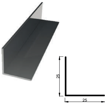
KALIP NO 4125 Kg / m: 0,159
