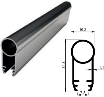
KALIP NO 4120 Kg / m: 0,313
