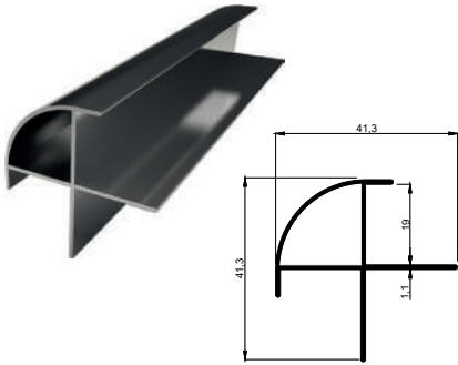
KALIP NO 4075 Kg / m: 0,376
