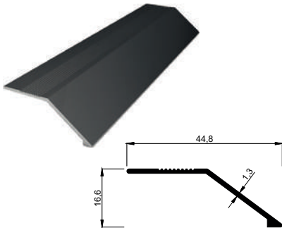
KALIP NO 4111 Kg / m: 0,177
