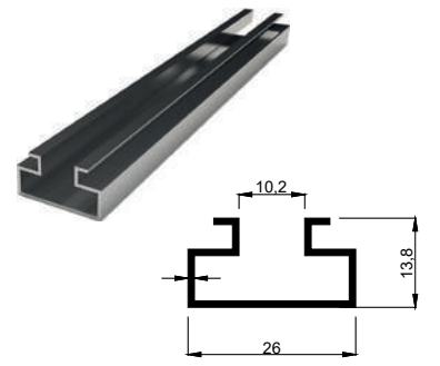
KALIP NO 4080 Kg / m: 0,192
