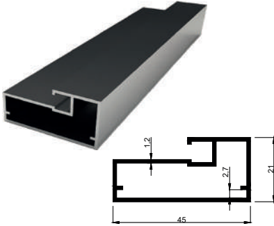
KALIP NO 4099 Kg / m: 0,449
