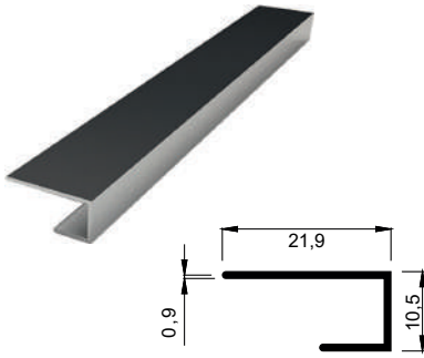
KALIP NO 4108 Kg / m: 0,097
