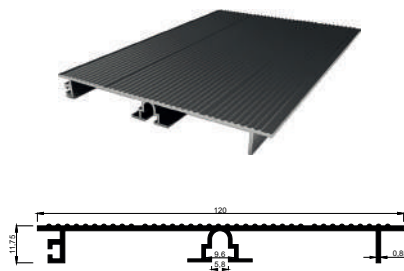
KALIP NO 4046 Kg / m: 0,473
