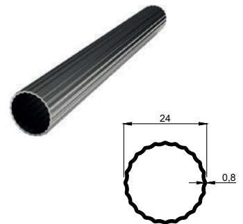
KALIP NO 4104 Kg / m: 0,159
