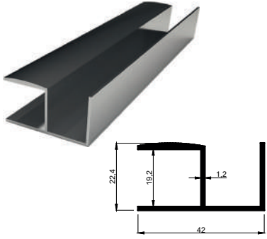
KALIP NO 4000 Kg / m: 0,363
