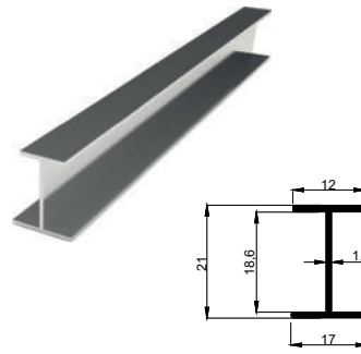
KALIP NO 4051 Kg / m: 0,148
