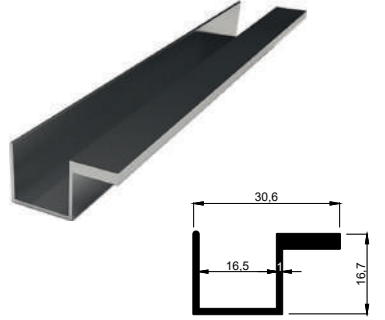
KALIP NO 4008 Kg / m: 0,265
