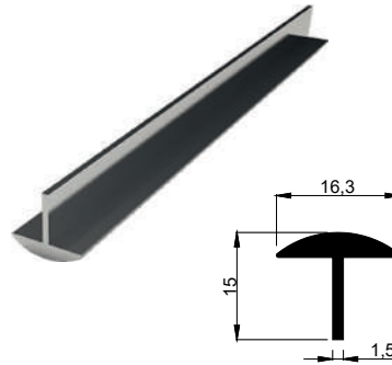
KALIP NO 4054 Kg / m: 0,145
