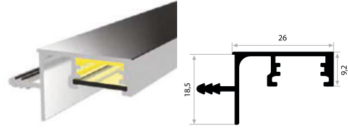
KALIP NO 6015 Kg / m: 0,306
