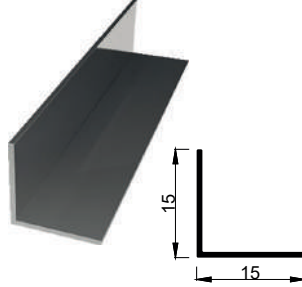
KALIP NO 4123 Kg / m: 0,087
