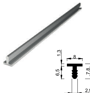
KALIP NO 4057 Kg / m: 0,066
