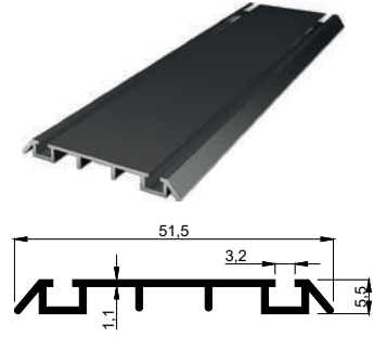
KALIP NO 4083 Kg / m: 0,263
