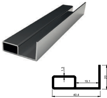
KALIP NO 4015 Kg / m: 0,240
