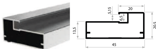
KALIP NO 2006 Kg / m: 0,431
