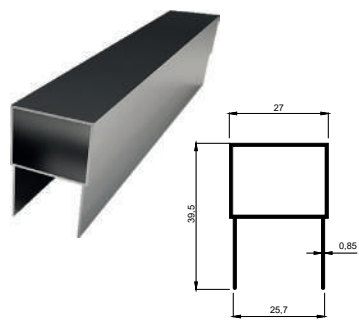
KALIP NO 4115 Plise Kasa Sineklik Kg / m: 0,300
