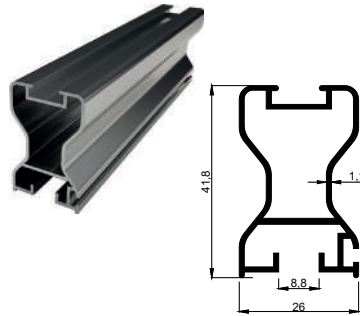
KALIP NO 4088 Kg / m: 0,522
