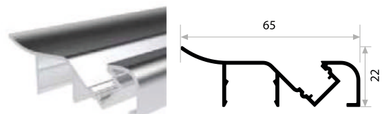
KALIP NO 6010 Kg / m: 0,541
