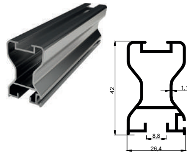
KALIP NO 4089 Kg / m: 0,481
