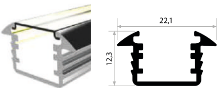
KALIP NO 6007 Kg / m: 0,173
