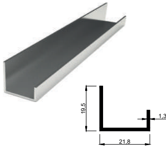
KALIP NO 4043 Kg / m: 0,175
