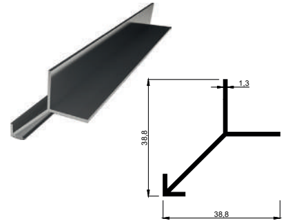
KALIP NO 4077 Kg / m: 0,265
