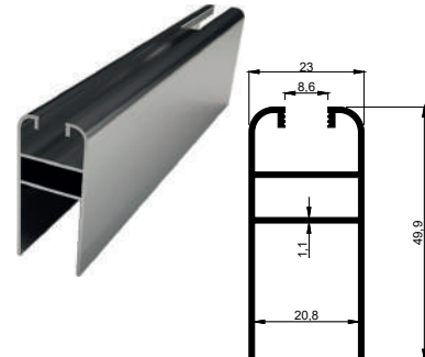
KALIP NO 4086 Kg / m: 0,479
