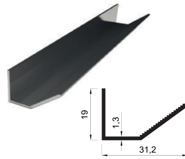
KALIP NO 4031 Kg / m: 0,184
