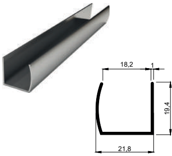
KALIP NO 4036 Kg / m: 0,155
