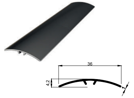
KALIP NO 4107 Kg / m: 0,117
