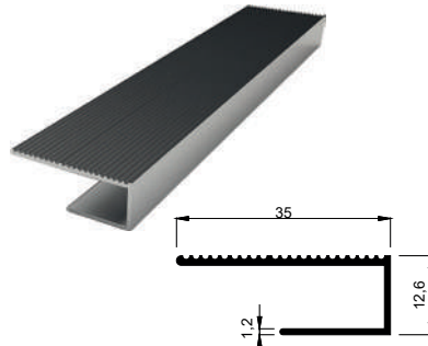
KALIP NO 4109 Kg / m: 0,174
