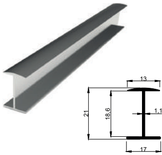
KALIP NO 4050 Kg / m: 0,141
