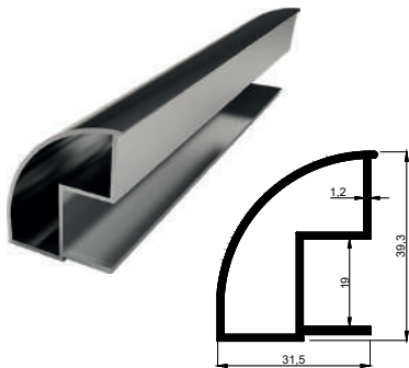
KALIP NO 4018 Kg / m: 0,482
