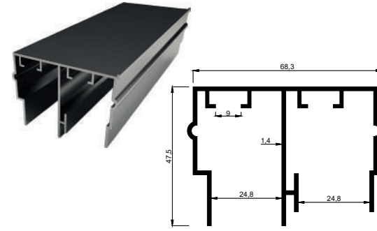
KALIP NO 4074 Kg / m: 0,950
