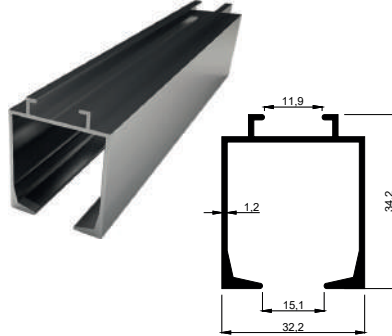
KALIP NO 4071 Kg / m: 0,422
