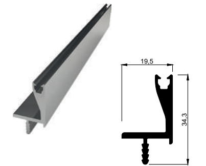
KALIP NO 4032 Kg / m: 0,382
