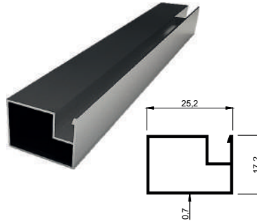
KALIP NO 4112 17x25 Sineklik Kg / m: 0,165
