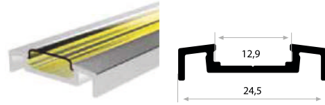
KALIP NO 6004 Kg / m: 0,128
