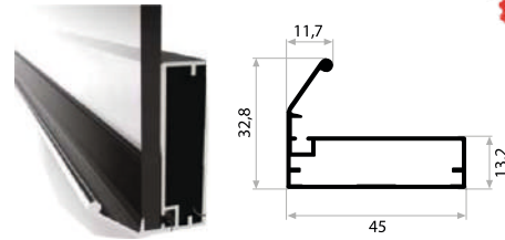
KALIP NO 2002 Kg / m: 0,490
