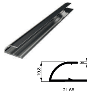
KALIP NO 4092 Kg / m: 0,115
