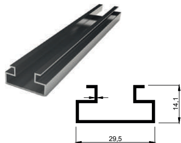
KALIP NO 4078 Kg / m: 0,231
