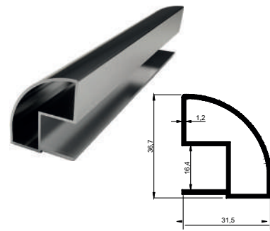
KALIP NO 4017 Kg / m: 0,465
