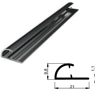
KALIP NO 4090 Kg / m: 0,107
