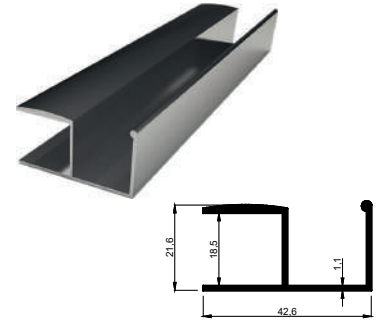
KALIP NO 4002 Kg / m: 0,351
