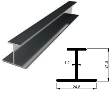
KALIP NO 4047 Kg / m: 0,172
