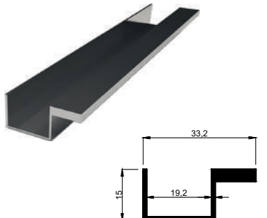
KALIP NO 4011 Kg / m: 0,256
