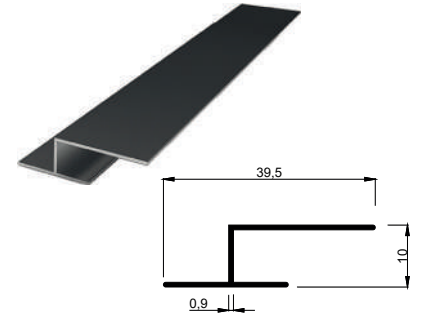
KALIP NO 4110 Kg / m: 0,148
