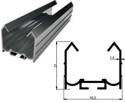
KALIP NO 4070 Kg / m: 0,660
