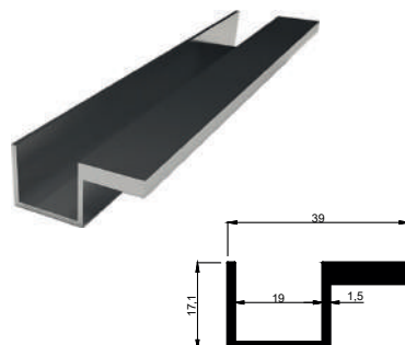
KALIP NO 4010 Kg / m: 0,446
